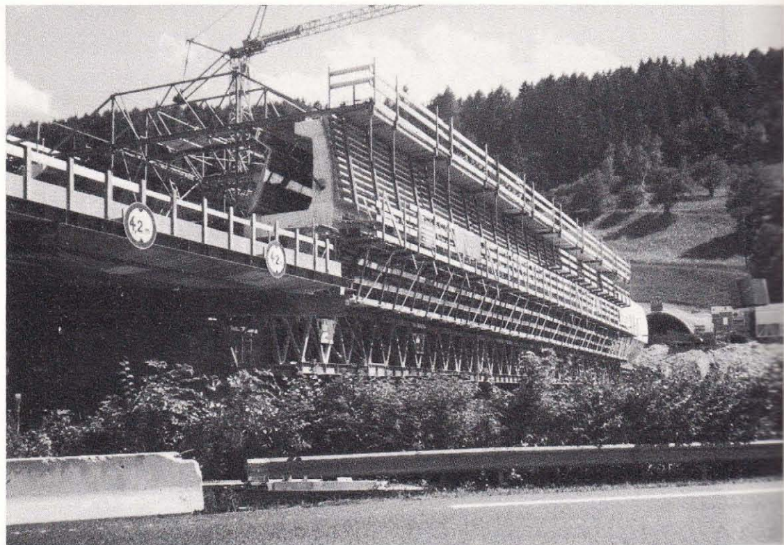
Tirols größte Baustelle ist die Bahnumfahrung Innsbrucks mit der Hochbrücke über Autobahn und Inn, im Volksmund „Sautrog“ genannt (Bauzustand vom Juni 1991). Foto Archiv
